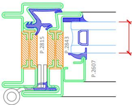
Inward Opening Door
